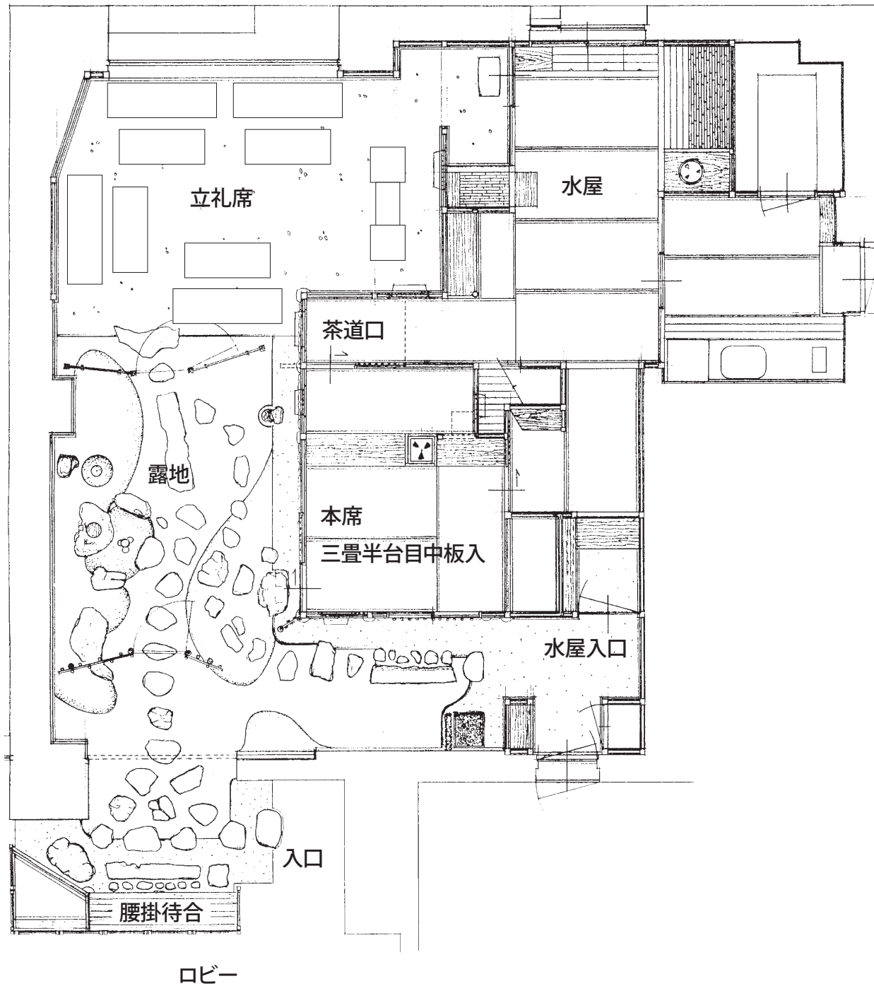
別紙 1 - 1 助庵平面図
