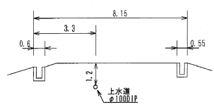
⑤ 断面図
