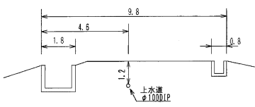
④ 断面図
